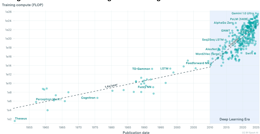
Abbildung 2-1: KI-Modelle und Trainingsrechenleistung
